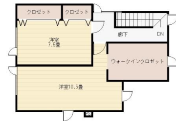
2階平面図
