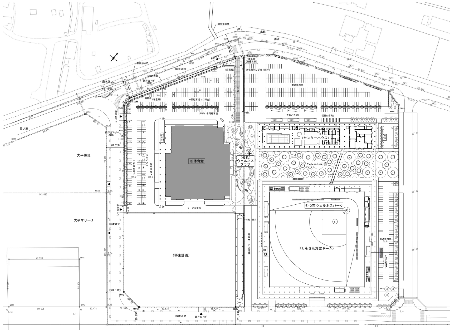
■配置図 1:1,500
