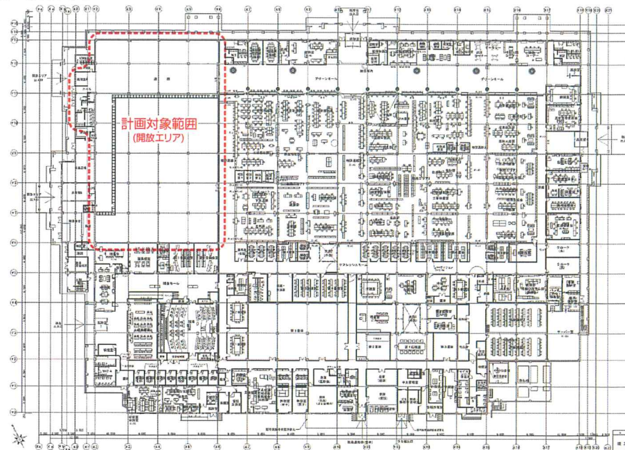
■現況1階平面図
