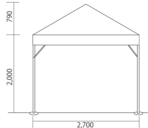
立面図
