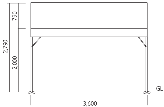
側面図
