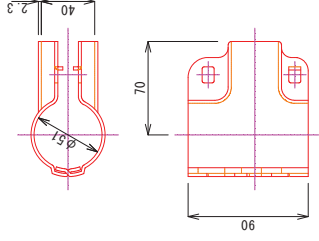
端ジョイント S=1:2
