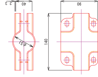
中間ジョイント S=1:2
