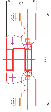
コーナー・傾斜ジョイント S=1:2
