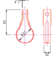
端バンド S=1:2
