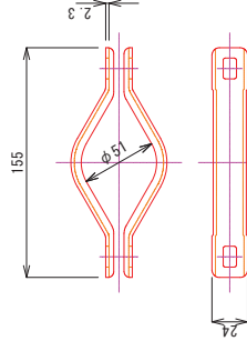
中間バンド S=1:2
