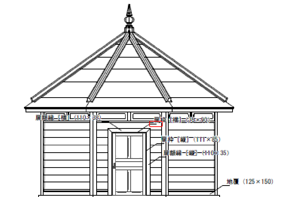
南立面図
