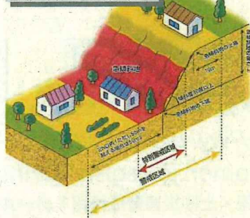
急傾斜地の崩壊
