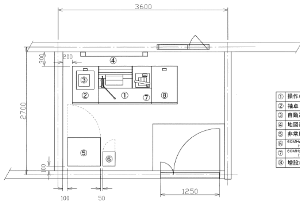
放送室 機器配置図(最終)
